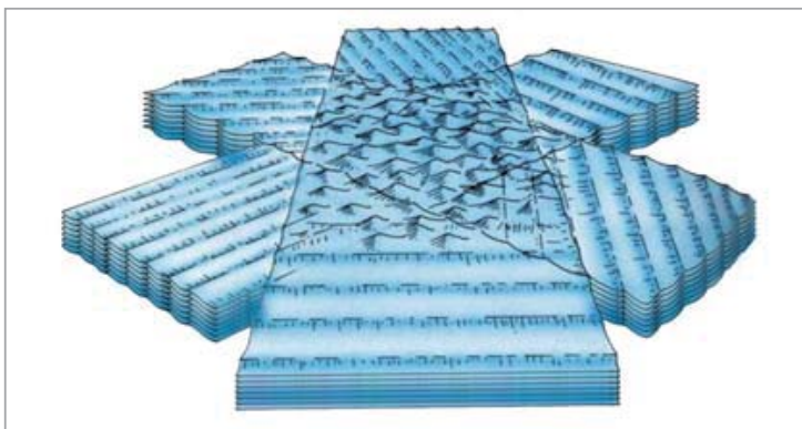
► Sóng ngầm tại giao diện của hai tầng nước có mật độ khác nhau. Một tầng dày đặc (tầng bên dưới), một tầng kia ít đậm đặc hơn (trên). (Hải dương học, Gross, trang. 204).
