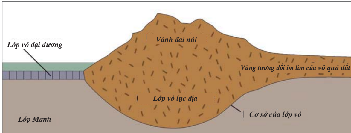
► Sơ đồ vỏ trái đất
