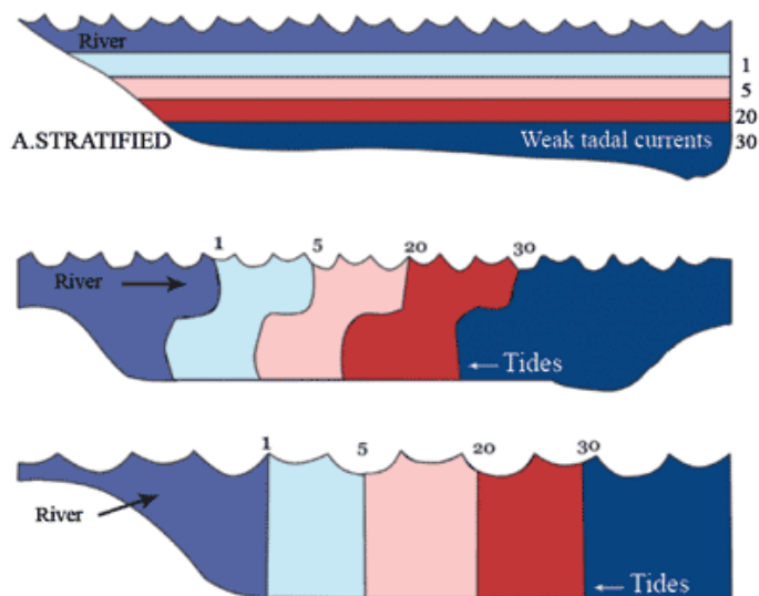
Tri typy stratifikácie salinity v pobrežných vodách: stratifikovaná; čiastočne zmiešaná a plne zmiešaná.
