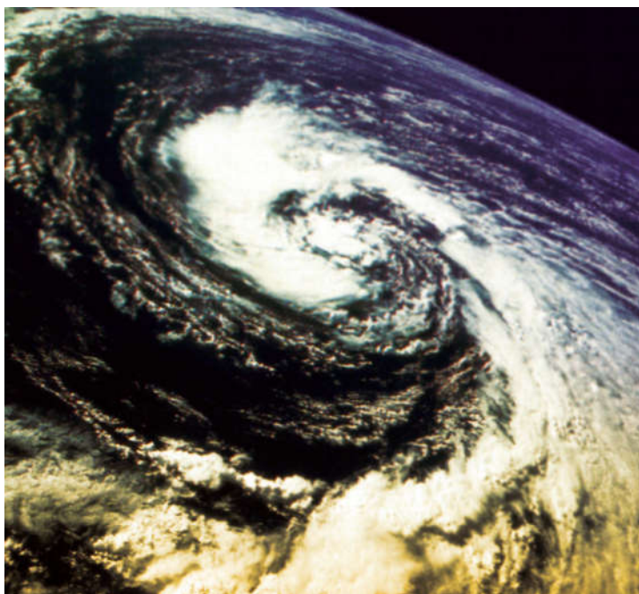
► Слика атмосфере која представља облаке и ветрове.
