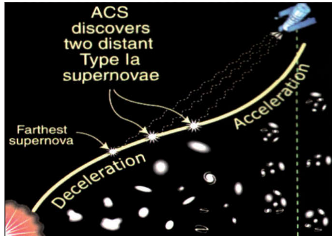
► Слика показује ширење универзума.
