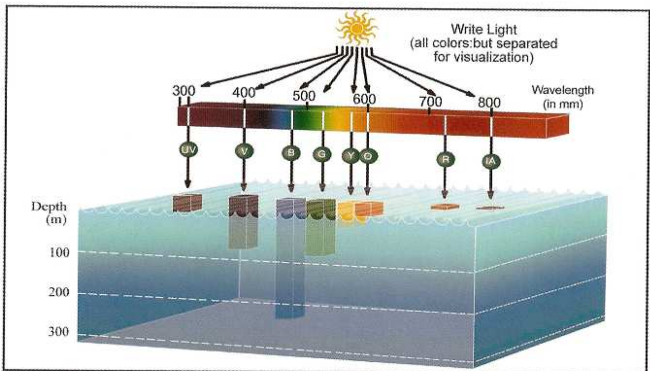
Dieses Diagramm zeigt die Tiefe, bis zu welcher das Licht klares Ozeanwasser durchdringt. Weil rotes Licht stark absorbiert wird, hat es die oberflächlichste Durchdringungstiefe; blaues Licht hat die tiefste Durchdringungstiefe. (Angewandte Optik, Vol. 20 (177) Smith, R.C. und K.S. Baker. 1981) Siehe auch offizielle NASA Webseite.
