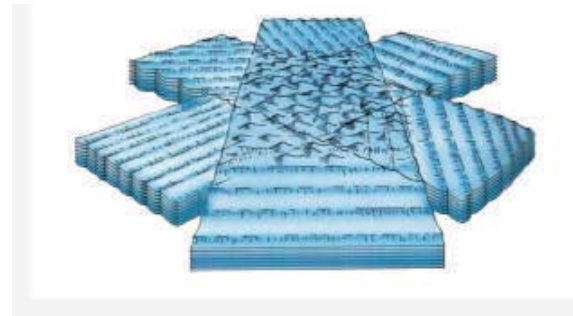
Les vagues internes à l'interface entre deux couches d'eau de densités différentes. L'une est dense (celle du bas), l'autre est moins dense (celle du haut). (Oceanography, Gross, p. 204)
