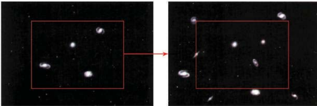
Cette image montre que les distances entre les galaxies ou les amas de galaxies sont en constante augmentation et que, par conséquent l'univers est en expansion.
