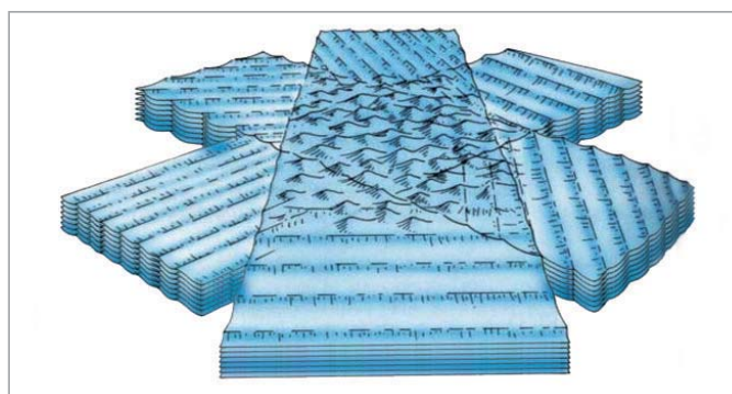
► Sisäiset aallot ja meren sekoittuminen. (Oceanography, Chris Garrett. Katso myös: http://www.nature.com/nature/journal/v422/n6931/full/422477a.html )
