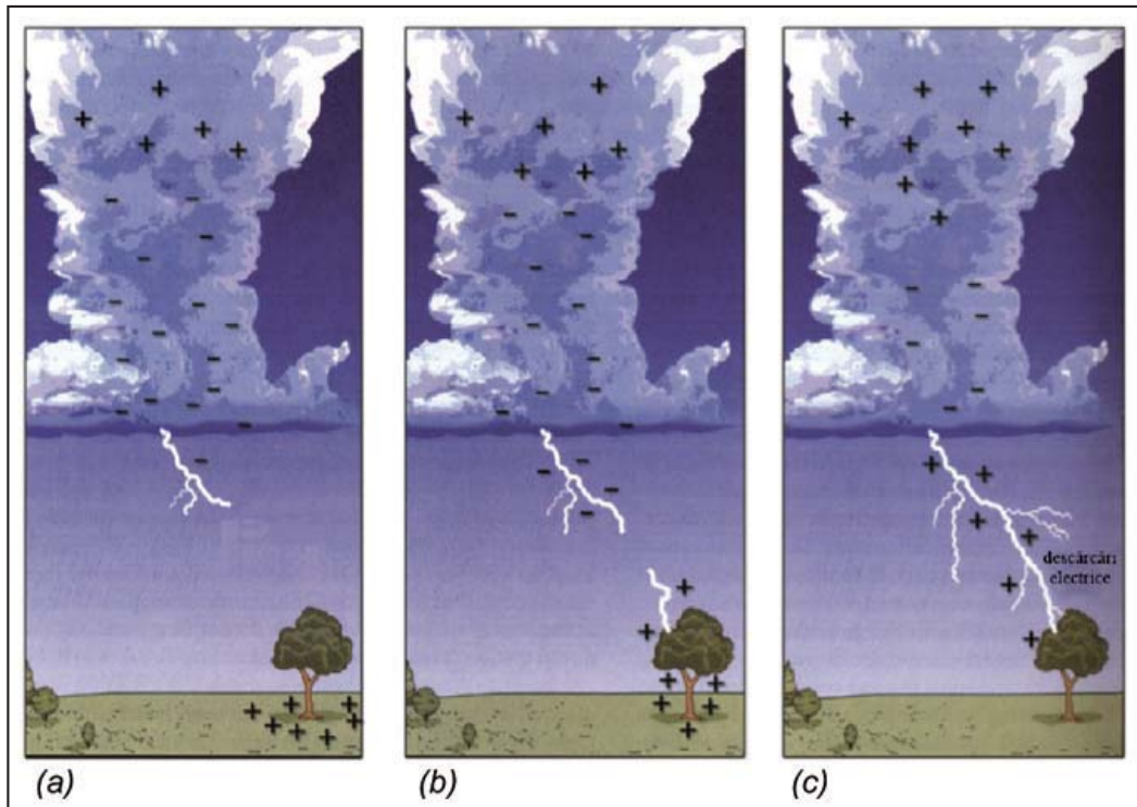
Kaava haarautuvasta salamasta. (a) Pilven alaosassa oleva negatiivinen varaus suurenee tarpeeksi päihittääkseen ilmanvastuksen ja kehittää ”johtajan” eli esisalaman, joka osoittaa kohti maata. (b) Positiiviset varaukset tulevat maasta ylös kohti. (c) Alas tulevat negatiiviset varaukset kohtaavat ylös suuntaavat positiivisten varaukset ja voimakas sähkövirta nimeltä pääsalama kantaa positiiviset varaukset pilveen.
