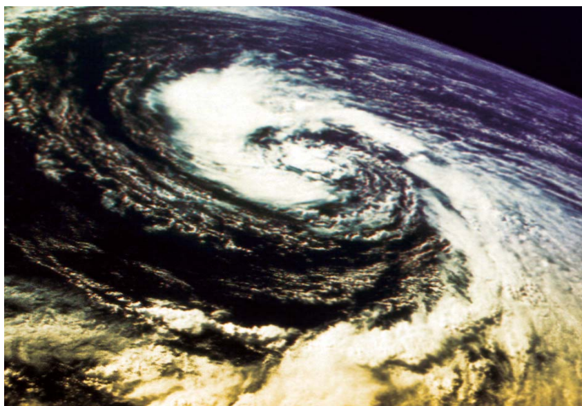
► Imakehä ja sen pilvet ja tuulet.
