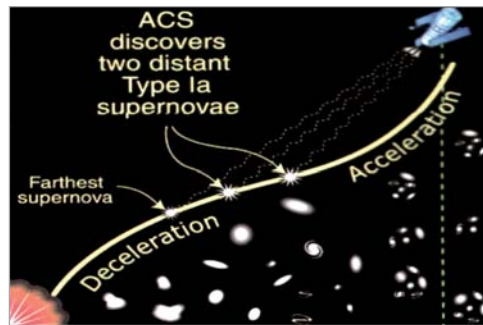
► Dit figuur laat zien dat het heelal uitdijt. De zogenaamde "Big Bang" theorie.
