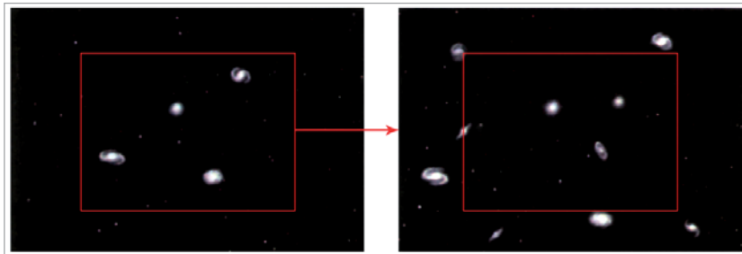
► Deze foto laat zien dat de afstanden tussen sterrenstelsels of clusters van sterrenstelsels voortdurend toeneemt en dat daarom het heelal uitdijt.
