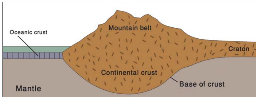
► Dit diagram toont de wortels van een berg. Sommige van deze wortels kunnen zestig kilometer lang zijn.
