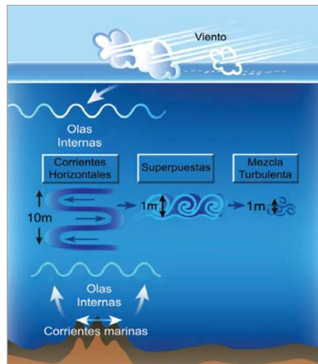
► Interne golven van de oceaan die zich mengen. (Oceanography, Chris Garrett)
