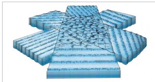
► Interne golven op grensvlak tussen twee lagen van water met verschillende dichtheden. De ene is zwaar (de onderste), de andere heeft een mindere dichtheid (de bovenste). (Oceanography, bruto, p. 204).
