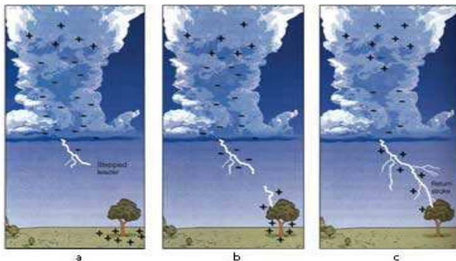
Model rozvětveného blesku. (a) Záporný náboj koncentrovaný ve spodní části oblaku zesílí natolik, že jej už izolující vrstva vzduchu neudrží a vytvoří se vůdčí výboj blesku mířící k zemi. (b) Vstřícný výboj s kladným nábojem vychází nejčastěji z vyvýšených míst na zemi. (c) Dochází ke spojení záporně nabitého vůdčího a kladně nabitého vstřícného výboje a vzniká mohutný elektrický proud, tzv. hlavní výboj blesku, kterým všechny náboje v oblaku zaniknou.
