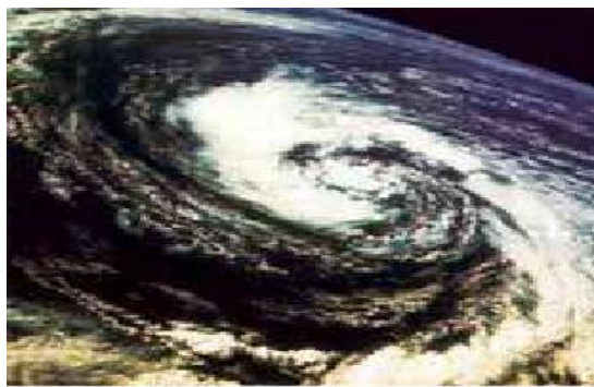
Slika atmosfere uključujući oblake i vjetrove.
