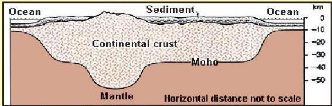
चित्र ७ : पर्वतका गहिरो जराहरू (Earth, Press & Siever, पृ स ४१३)
