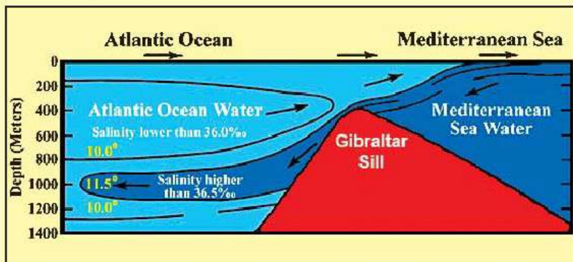
चित्र १३ : जिब्राल्टरको सिलमाथिबाट भूमध्यसागरको पानीको अट्लान्टिक महासागरमा प्रवेश। तापमान सेन्टिग्रेडमा। ("Marine Geology," Kuenen, पृ. ४३)
