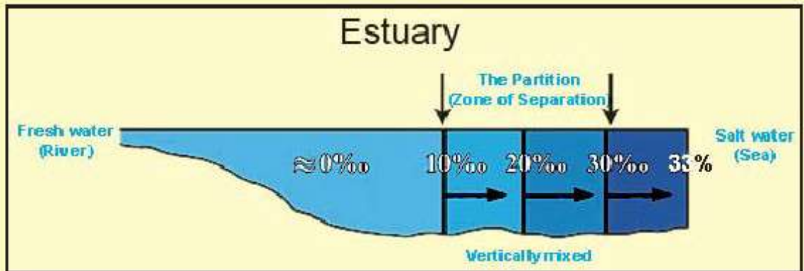
चित्र १४ : मुहान (Estuary) को नूनिलोपना देखाउने रेखीय चित्रण । यसमा ताजा पानी र नूनिलो पानी बीचको विभाजन-क्षेत्र (Zone of Separation) देखाइएको छ । ("Introductory Oceanography, Thrumann, पृ ३०१)
