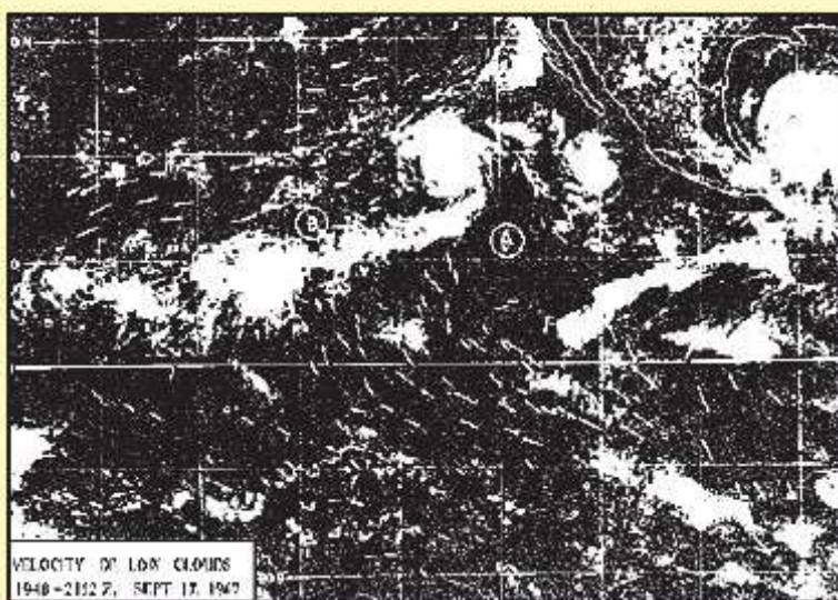
चित्र १७ : भू-उपग्रहद्वारा खिचिएको यस चित्रमा बादलहरू जमाव-क्षेत्रहरू B, C, D तिर गतिमान देखिन्छन्। तीरको चिन्हले यस गतिको दिशा देखाउँछ। ("The Use of Satellite Pictures in Weather Analysis and Forecasting: Anderson & Others, पृ ११८)
