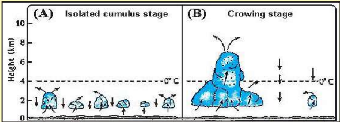
चित्र १९ : (A) Cumulus बादलका स-साना टुक्राहरू (B) जोडिएर बनेको ठूलो बादल। पानीका थोपाहरू बिन्दु (.) द्वारा दर्शाइएका छन्। ("The Atmosphere," Amthes & Others, पृ २६९)
