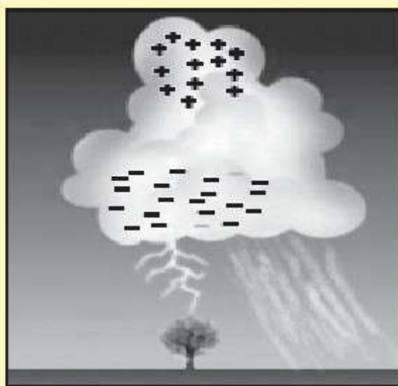
चित्र २२ : Negative Charge भूइतिर बज्रपातको रूपमा भन्दै ।
