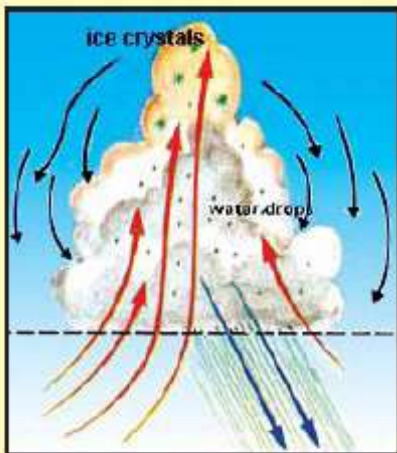
चित्र २० : एउटा Cumulonimbus बादल। ("Weather and Climate," Bodin पृ १२३)।
