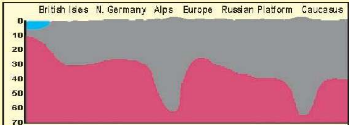
चित्र ८ : पर्वतका जमीनमा गाडिएका चुकुल (Peg) जस्ता जराहरू (Anatomy of the Earth Cailleux, पृ स २२०)
