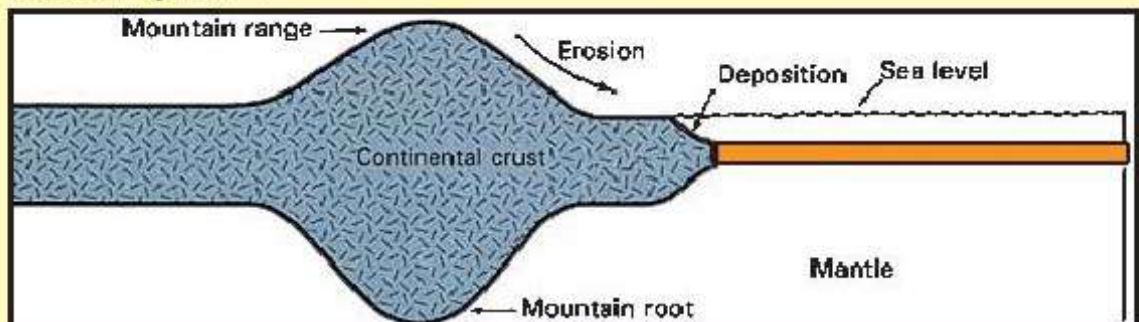
चित्र ९ : गहिरो जराहरूको कारणले चुकुल (Peg) जस्तो आकार लिएको पर्वतहरू देखाउने अर्को चित्र ("Earth Science" Tarbuck & Lutgens, पृ स १५८)
