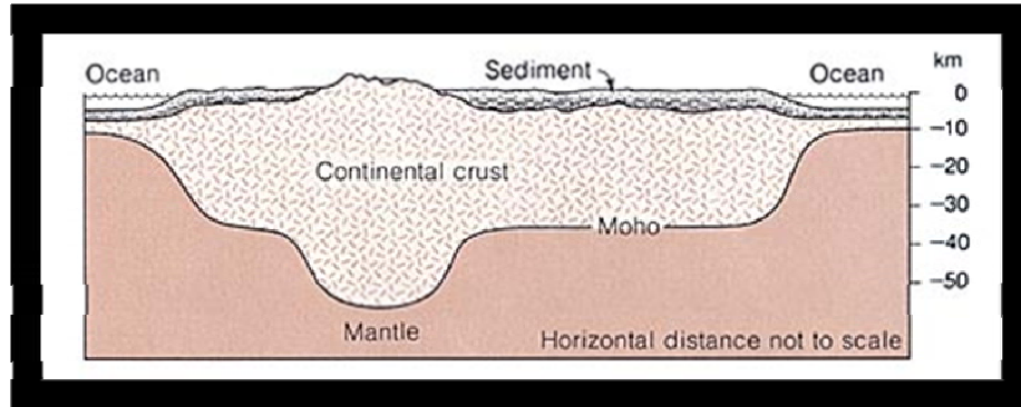
7: Munții au rădăcini sub pamant (1)
