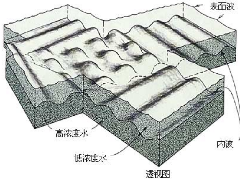
图 16：两层不同密度水域之间的内海。一层较密（下层），另一层较松（上层）。(Oceanography [海洋学]，作者葛雷斯 (Gross)，第 204 页。)
