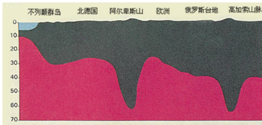
图 8： 截面示意图。 状似木桩的山有植入土地的深根。（Anatomy of the Earth [地球结构]，作者西里士 (Cailleux)，第 220 页。）
