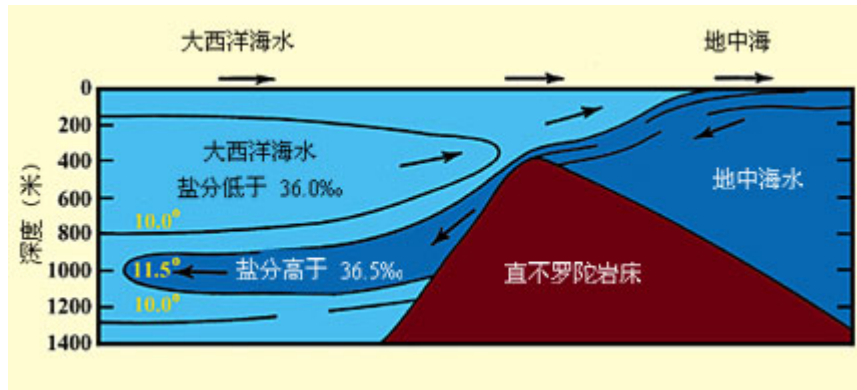
图 13：地中海的海水，从直布罗陀海底山脊的上方进入大西洋后仍能保持其本身温暖、含盐及低密度的特质，是因为这条界限将它们隔开。温度以摄氏表示 (C°)。(Marine Geology [海洋地质学]，作者昆宁 (Kuenen)，第 43 页，稍有改动。
