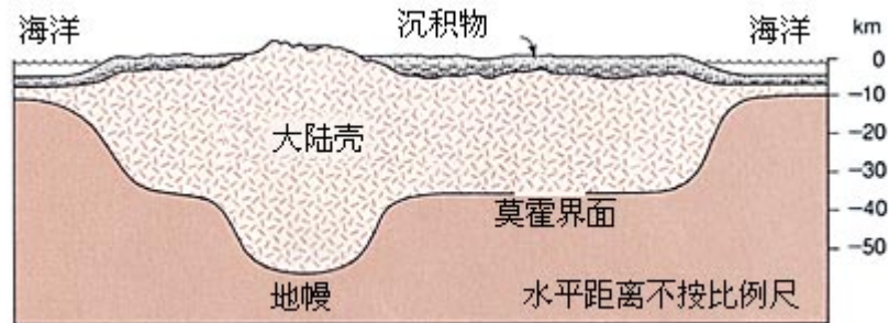
图 7：山在地表下有深根。(Earth [地球]，作者普雷斯 (Press) 与西瑞尔 (Siever)，第 413 页。)
