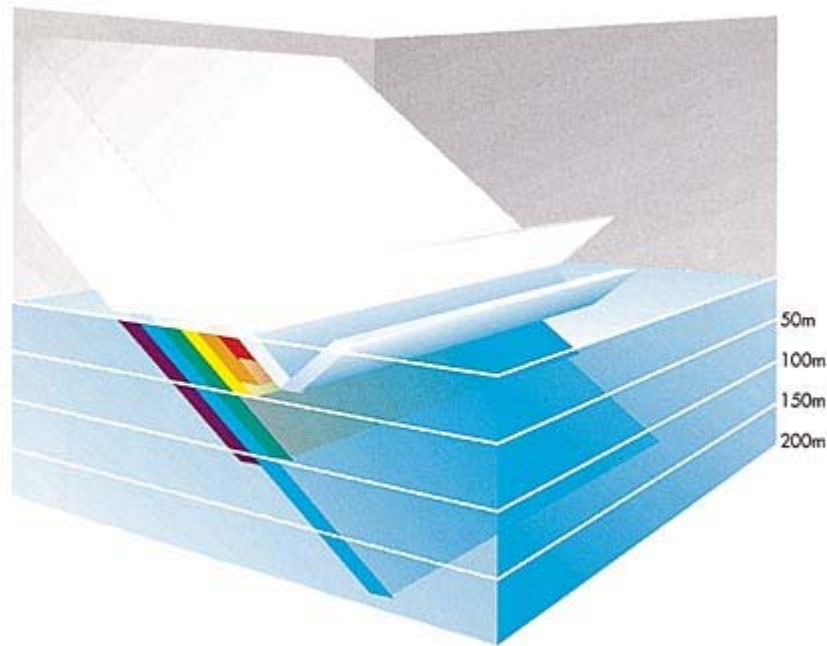
图 15：海平面会反射 3% 到 30% 的阳光。因此除了蓝光之外，光谱中的七种色彩几乎会在前 200 米逐一被吸收。 （ Oceans [海洋]，作者爱尔德 (Elder) 与巴内特 (Pernetta)，第 27 页。）
