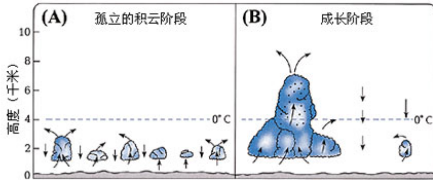
图 19: (A) 分离小块云片 (积云)。 (B) 当小型云结合在一起, 大型云的上升气流随即增加, 云也将往上堆积。·代表雨滴。(The Atmosphere [大气], 作者恩西斯 (Anthes) 等, 第 269 页。)
