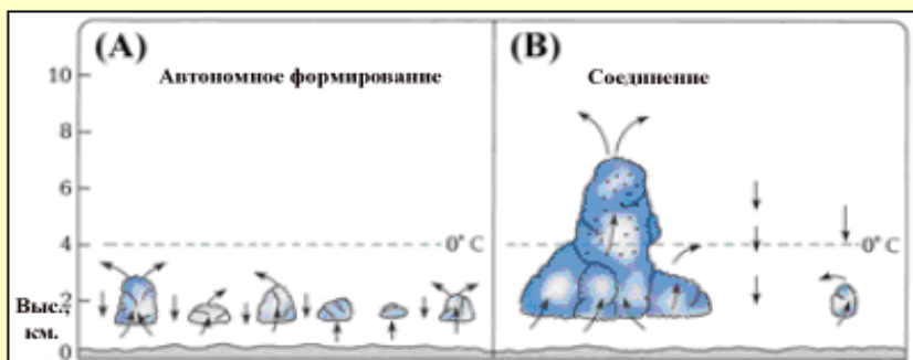
Рис. 19: (А) Отдельные маленькие облака (кучевая обл.). (В) Маленькие облака собираются вместе и восходящие потоки увеличивают облако, формируя его. Капли дождя обозначены •. (Атмосфера, Антес и др, р. 269.)
