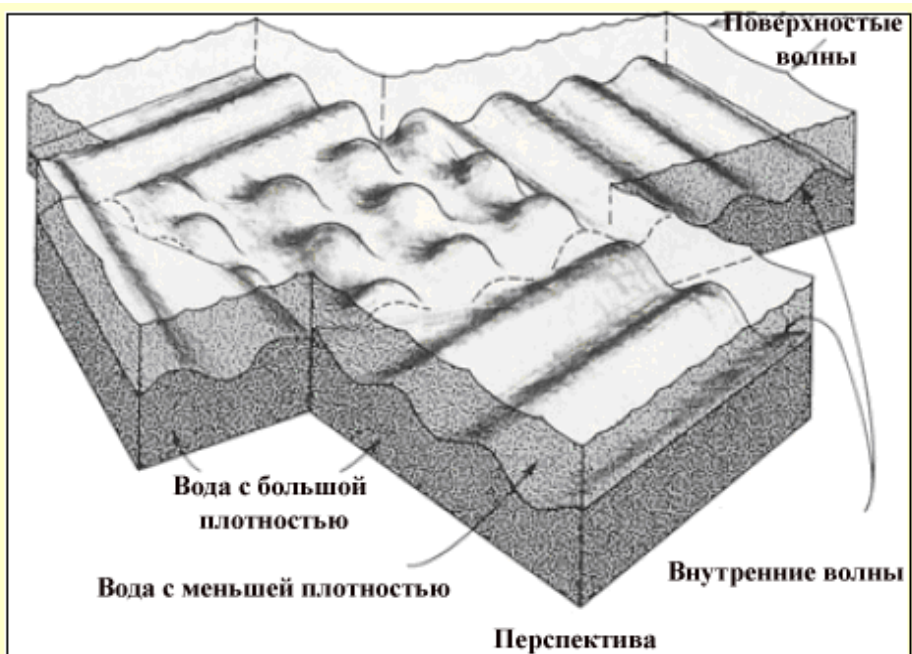
Рис. 16: Внутренние волны на границе раздела двух слоёв воды с разной плотностью. Один плотен (более низкий), другой менее плотен (верхний). (Океанография, Гросс, стр. 204.)
