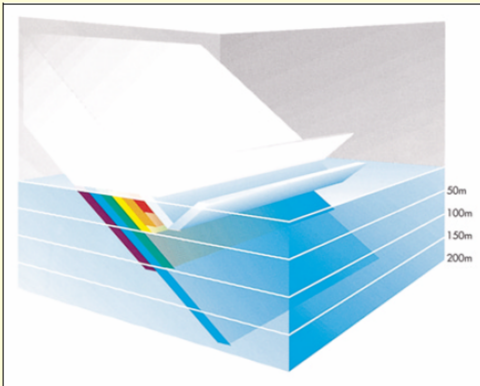
Рис. 15: От 3 до 30 процентов солнечного света отражается от морской поверхности. Затем почти все семь цветов светового спектра поглощаются один за другим в первых 200 метрах, кроме синего света. (Океаны, Эльдер и Пернетта, стр.27)
