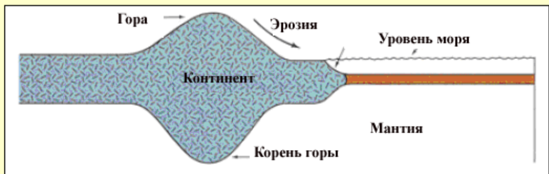
Рис. 9: Другая иллюстрация показывающая сходство гор с клиньем из-за их глубоких корней. ("Наука о Земле", Тарбок и Латдженс, стр. 158.)
