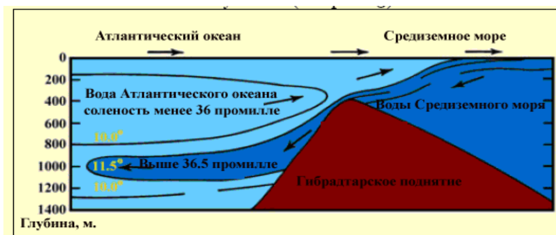
Рис. 13: Вода Средиземного моря, впадающая в Атлантику через Гибралтарский пролив сохраняет свои температуру, солёность и плотность, из-за барьера, разделяющего их. Температуры указаны в градусах Цельсия (С°). (Морская Геология, Кьунен, стр. 43, с небольшой поправкой.)
