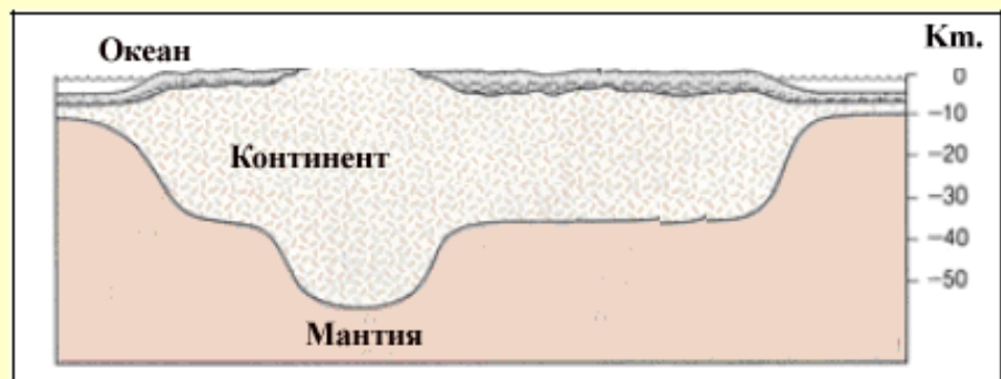
Рис. 7: Горы имеют глубокие корни под землёй ("Земля", Пресс и Сьювер, стр.413.)
