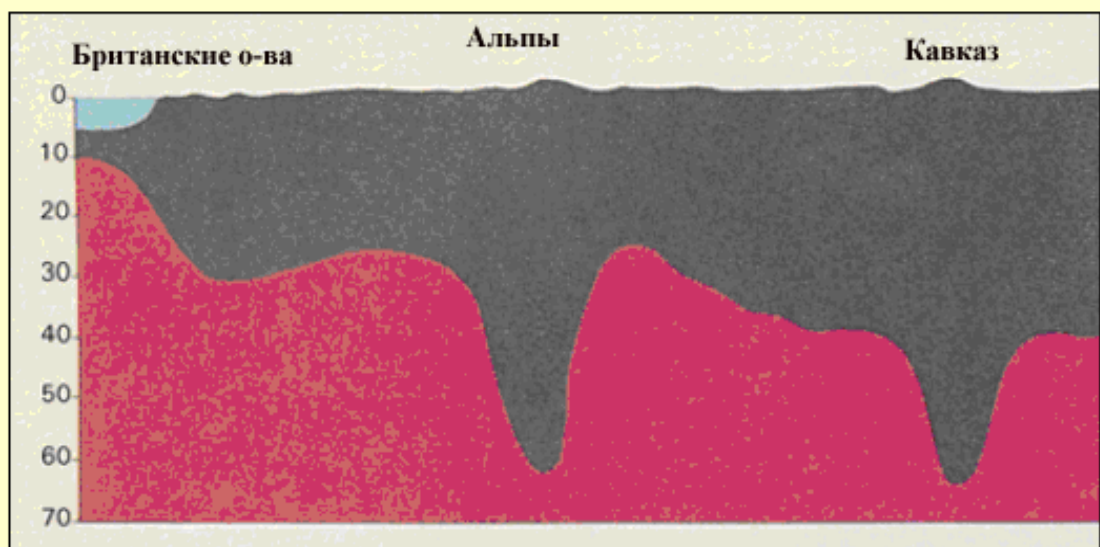
Рис. 8: Схематический разрез. Горы, подобно клиньям, имеют глубоко уходящие в землю корни. ("Анатомия Земли", Кайллюкс, стр. 220.)
