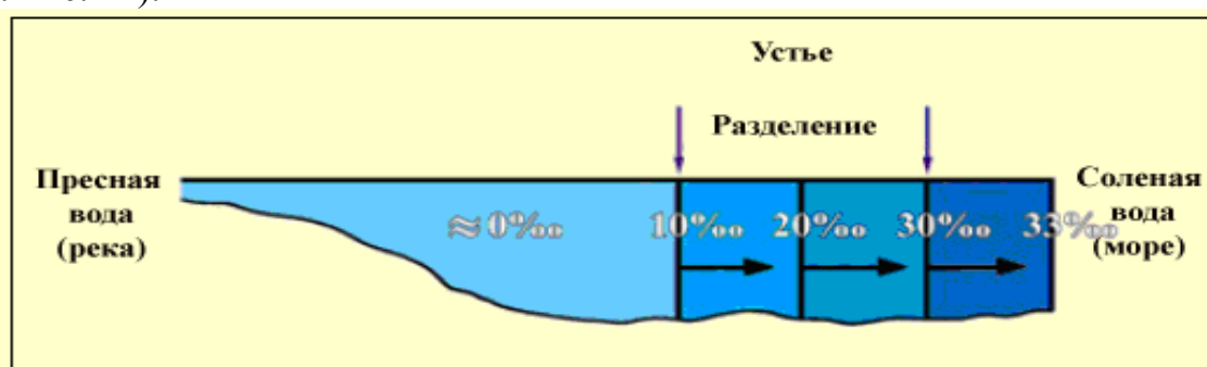
Рис. 14: Продольное сечение, показывающее солёность (в промилле) в устье. Мы можем видеть здесь преграду (зону разделела) между пресной и солёной водой. (Введение в Океанографию, Тармэн, стр. 301, с небольшим изменением.)
