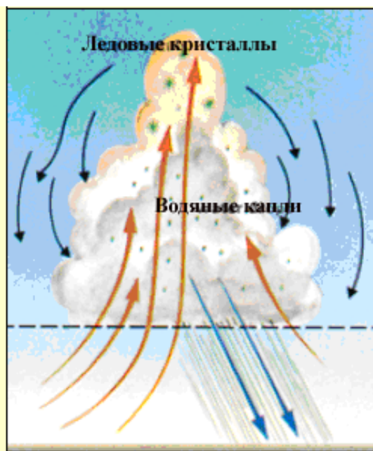
Рис. 20: Кучеводождевое облако. После образования облака, из него выпадает дождь. (Погода и климат, Бодин, стр.123.)
