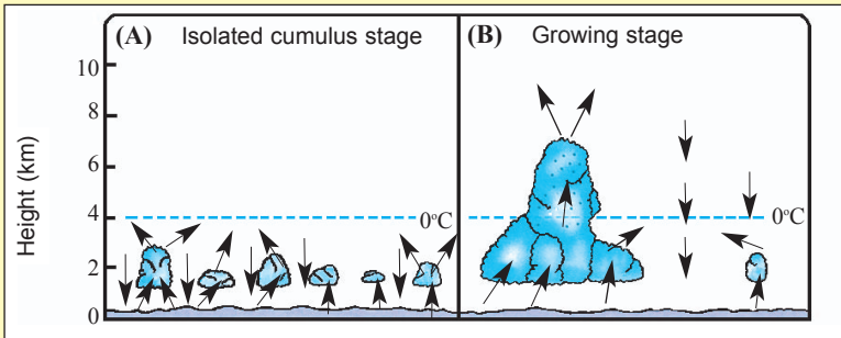
Фиг. 19. (А) Отделни малки облаци (кълбести облаци). (Б) Когато малките облаци се съберат заедно, вертикалните въздушни течения в по-големия облак нарастват, поради което облакът се издължава нагоре. Водните капки са отбелязани с •.
