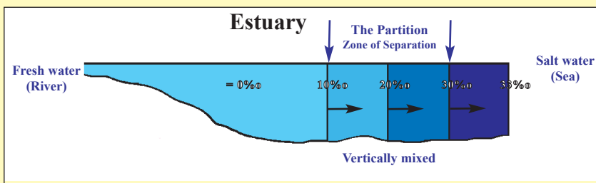
Фиг. 14. Надлъжен разрез, показващ солеността (в промили ‰) при устията на големи реки. Тук можем да видим зони на разделение между сладката и солената вода.
