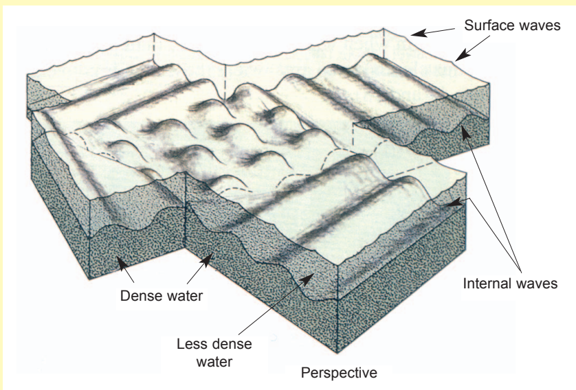
Фиг. 16. Вътрешногравитационните вълни при взаимодействие между два слоя вода с различна плътност. Първият (долният) е с по-голяма плътност, вторият (горният) е с по-малка плътност.
