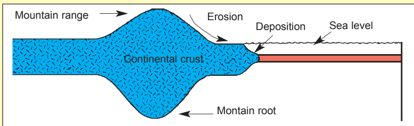
Фиг. 9. Планините придобиват формата на подпора заради дълбоките си корени.
