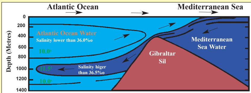
Фиг. 13. Водата от Средиземно море се влива в Атлантическия океан през Гибралтарския проток със своя характерна температура, соленост и плътност, заради разделящата ги бариера. Температурата е в градуси по Целзий (С°).
