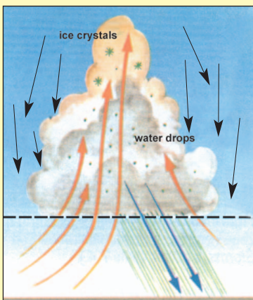
Фиг. 20. Кълбесто-дъждовен облак. След като облакът се издължи нагоре, дъждът започва да вали от него.
