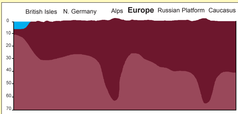
Фиг. 8. Схематичен разрез. Планините като подпори имат дълбоки корени в земната кора.
