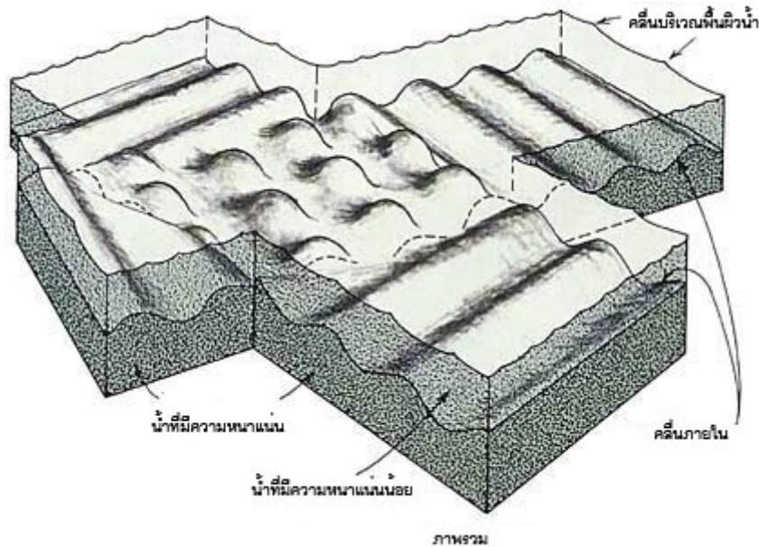
รูปที่ 16: คลื่นใต้น้ำบริเวณที่มีชั้นน้ำสองชั้นซึ่งมีความหนาแน่นต่างกันมาประสานกัน สายหนึ่งจะมีความหนาแน่นมากกว่า (สายที่อยู่ต่ำกว่า) ส่วนอีกสายหนึ่งจะมีความหนาแน่นที่น้อยกว่า (สายที่อยู่ด้านบน) (Oceanography ของ Gross หน้า 204)
