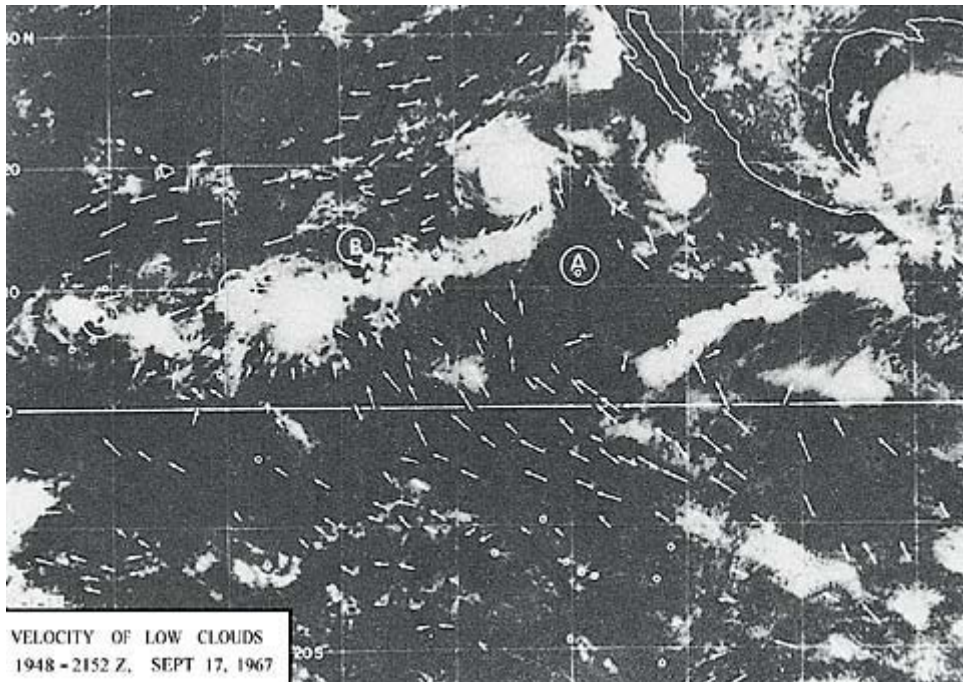
รูปที่ 17: จากภาพถ่ายดาวเทียมแสดงให้เห็นว่า กลุ่มเมฆต่างๆ กำลังเคลื่อนตัวไปข้างหน้าเพื่อไปบรรจบกันตรงบริเวณอักษร B, C และ D เครื่องหมายลูกศรจะบอกให้ทราบถึงทิศทางของกระแสลม ( The Use of Satellite Pictures in Weather Analysis and Forecasting ของ Anderson และคณะ หน้า 188) (คลิกที่รูปภาพเพื่อขยายใหญ่)
