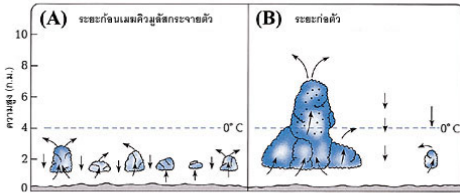
รูปที่ 19:(A) เมฆก้อนเล็กๆ ที่กระจัดกระจายกันอยู่ (เมฆฝนฟ้าคะนอง) (B) เมื่อเมฆก้อนเล็กๆ มารวมกัน กระแสอากาศไหลขึ้นในก้อนเมฆก็จะรุนแรงตามขึ้นไปด้วย จนกระทั่งก้อนเมฆมีขนาดใหญ่โตมาก จากนั้นก็กลั่นกลายกลับมาเป็นหยดน้ำ (The Atmosphere ของ Anthes และคณะ หน้า 269) (คลิกที่รูปภาพเพื่อขยายใหญ่)
