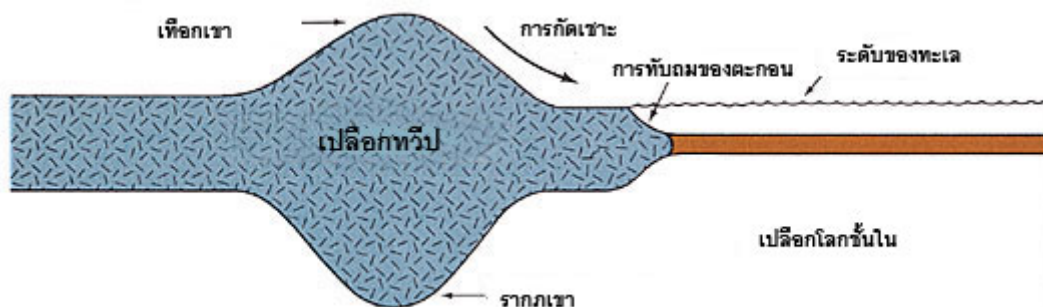
รูปที่ 8: ส่วนที่เป็นแผ่นผั่ง เทือกเขาที่มีรูปร่างเหมือนสลัก จะมีรากฝังแน่นอยู่ใต้พื้นดิน (Anatomy of the Earth ของ Cailleux หน้า 220) (คลิกที่รูปภาพเพื่อขยายใหญ่)
