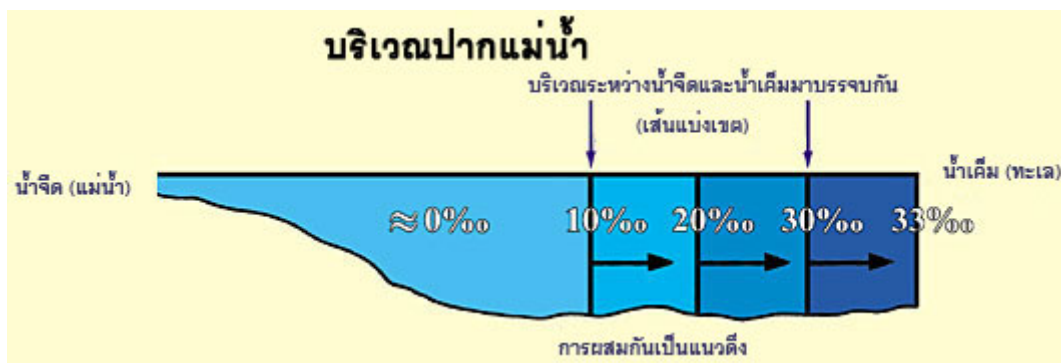
รูปที่ 14: ส่วนที่เป็นเส้นตรง แสดงให้เห็นถึงความเค็ม (ส่วน ต่อ หนึ่งในพันเปอร์เซ็นต์) ในบริเวณปากแม่น้ำ เราจะเห็นการแบ่งเขต (เขตการแบ่งแยก) ที่กั้นระหว่างน้ำจืดกับน้ำเค็ม ( Introductory Oceanography ของ Thurman หน้า 301 ฉบับปรับปรุงเพิ่มเติมเล็กน้อย) (คลิกที่รูปภาพเพื่อขยายใหญ่)
