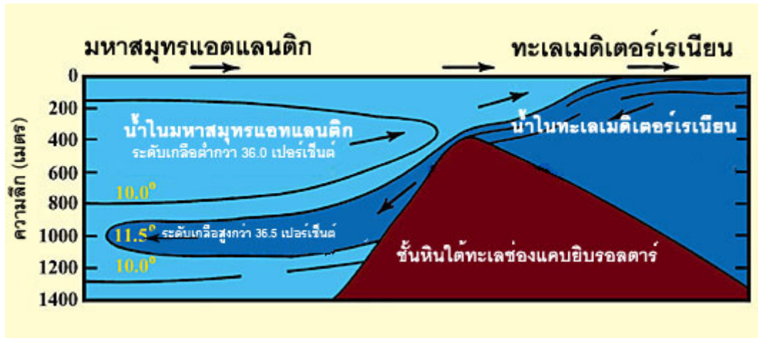
รูปที่ 13: น้ำจากทะเลเมดิเตอร์เรเนียนขณะที่หนุนเข้าไปในมหาสมุทรแอตแลนติกโดยผ่านทางสันดอนยิบรอลตาร์ ซึ่งจะพาความอุ่น
