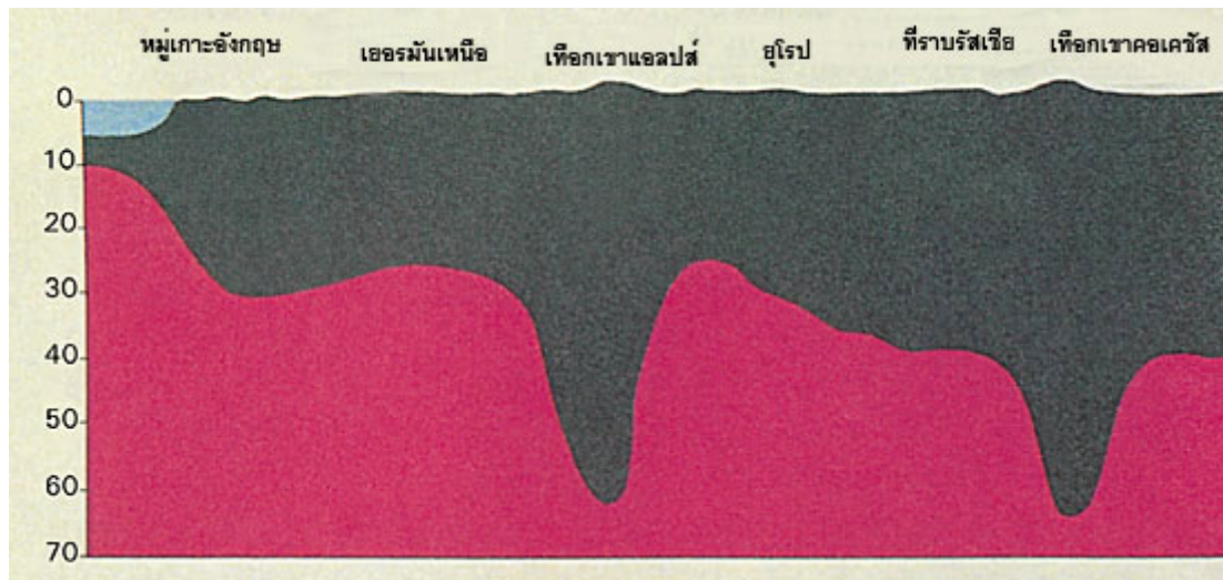
รูปที่ 8: ส่วนที่เป็นแผ่นผั่ง เทือกเขาที่มีรูปร่างเหมือนสลัก จะมีรากฝังแน่นอยู่ใต้พื้นดิน (Anatomy of the Earth ของ Cailleux หน้า 220) (คลิกที่รูปภาพเพื่อขยายใหญ่)
