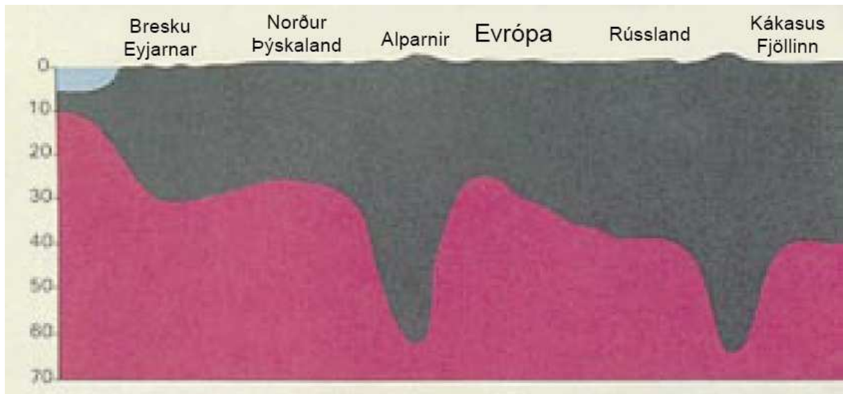
Skýringarmynd 8: Fjöllin eru eins og pinnar og hafa rætur djúpt undir yfirborði jarðar. („ Anatomy of the Earth ”, Cailleux, bls. 220.)
