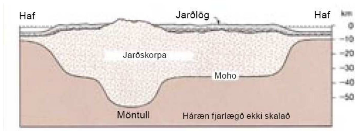
Skýringarmynd 7: Fjöll hafa rætur djúpt undir yfirborði jarðar ( Earth , Press og Siever, bls. 413.)
