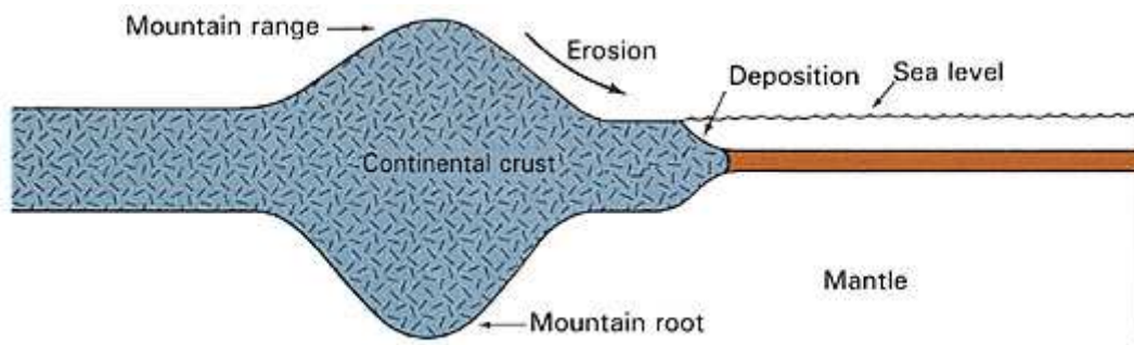
Skýringarmynd 9: Önnur skýringarmynd sem sýnir hvernig fjöll eru mynduð eins og pinnar, vegna djúpra róta undir fjöllum. („ Earth Science ”, Tarbuck og Lutgens, bls. 158.).
